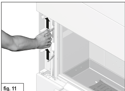
fig. 11 Tirer vers le haut les deux barres de verrouillage (gauche ou droite) (fig. 11).
