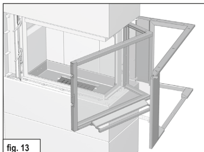
fig. 13 Porte du foyer ouverte avec cache du foyer ouvert (fig. 13).
