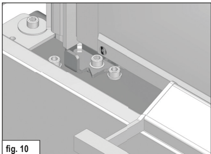
fig. 10 Dans cette position, la porte du foyer est bloquée et ne peut pas être soulevée (fig. 10).
